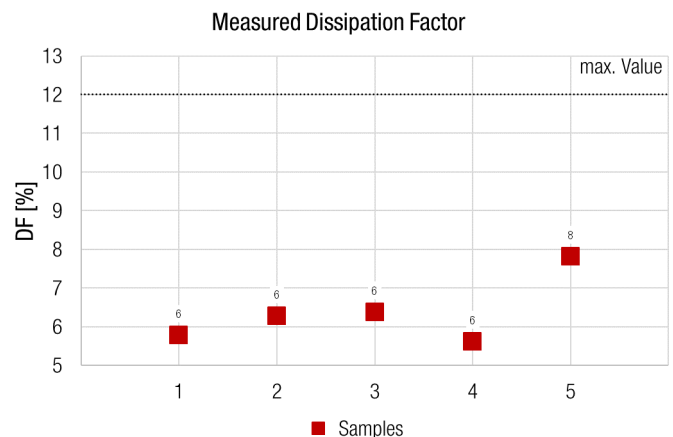
Abbildung 10: Verlustfaktor nach fünf Jahren Lagerung von fünf Mustern. Der maximal spezifizierte DF beträgt 12 % (Aluminium-Polymer-Kondensator)
