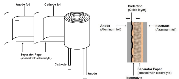
Abbildung 2: Aufbau eines Elektrolytkondensators
