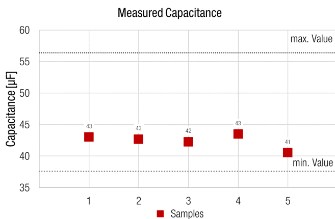
Abbildung 8: Kapazität nach fünf Jahren Lagerung von fünf Mustern. Die Nennkapazität beträgt 47µF (Aluminium Polymer-Kondensator)
