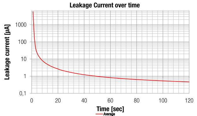
Abbildung 4: Durchschnittlicher Leckstrom von 10 Kondensatoren, gemessen über 2 Minuten.
