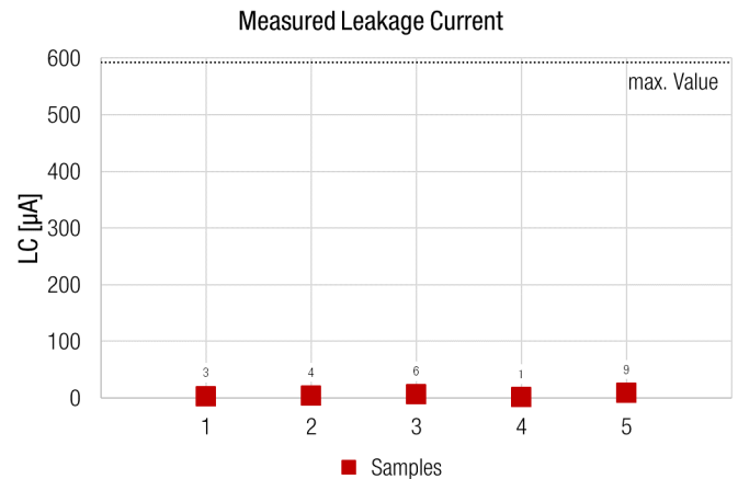
Abbildung 9: Leckstrom nach fünf Jahren Lagerung von fünf Mustern. Der maximal spezifizierte Leckstrom beträgt 559µA (Aluminium-Polymer-Kondensator)
