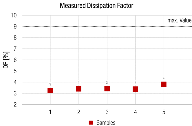
Abbildung 6: Verlustfaktor nach fünf Jahren Lagerung von fünf Mustern. Der maximal spezifizerte DF beträgt 9% (Aluminium-Elektrolytkondensator)
