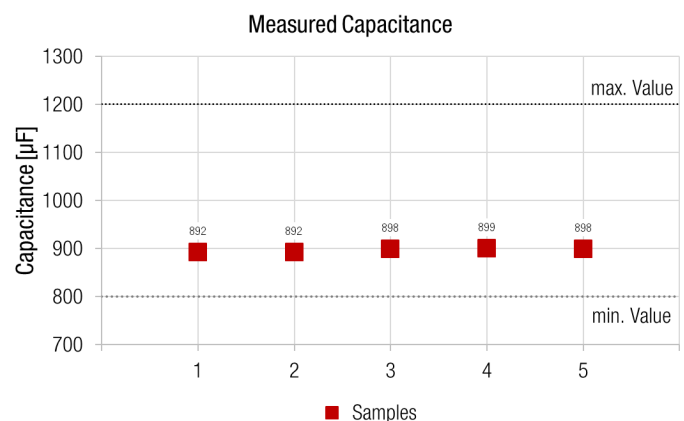
Abbildung 5: Kapazität nach fünf Jahren Lagerung von fünf Mustern. Die Nennkapazität beträgt 1000 \mu F (Aluminium-Elektrolytkondensator)
