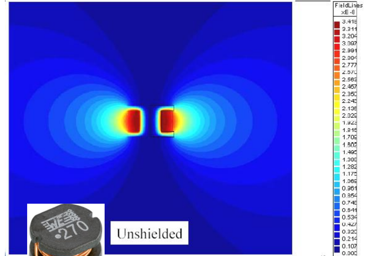
Ungeschirmte Drossel
