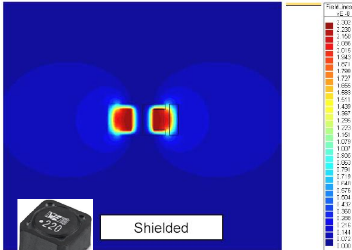
Geschirmte Drossel
