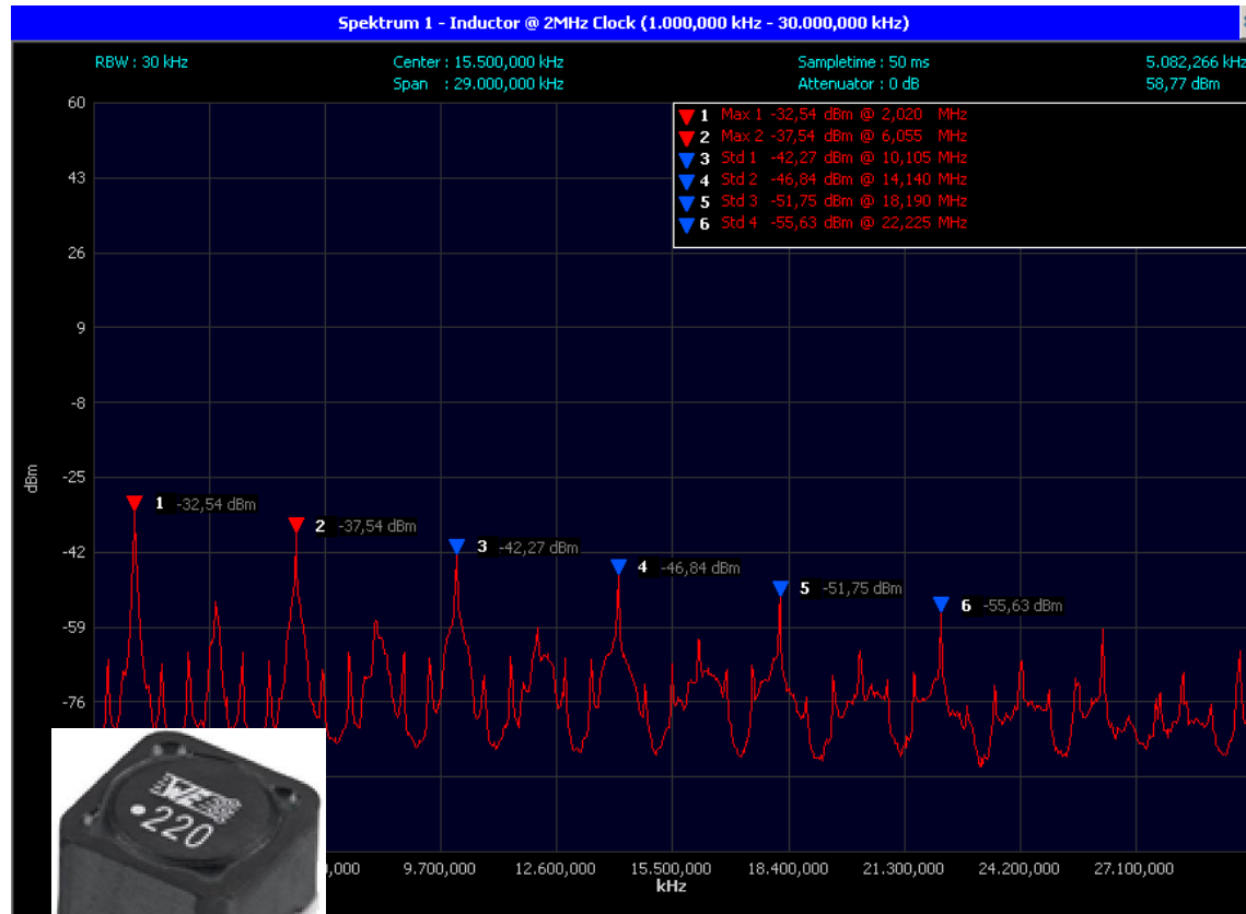
Geschirmte Drossel
