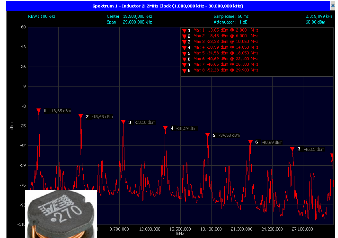
Ungeschirmte Drossel
