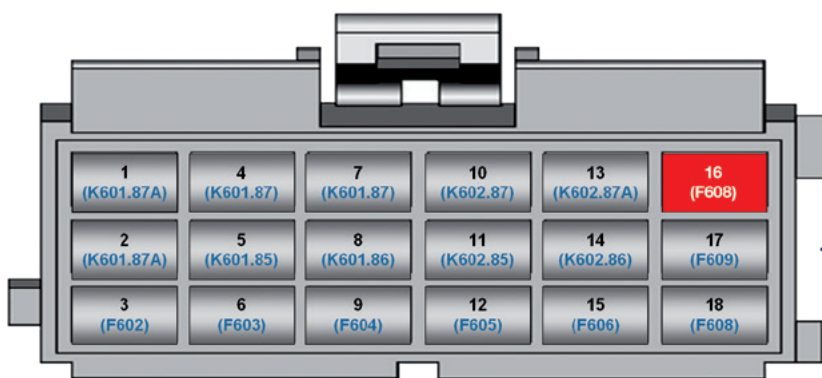
Steckverbinder (Buchse) für Kabelanschluss (Ansicht Kabeleingang)
