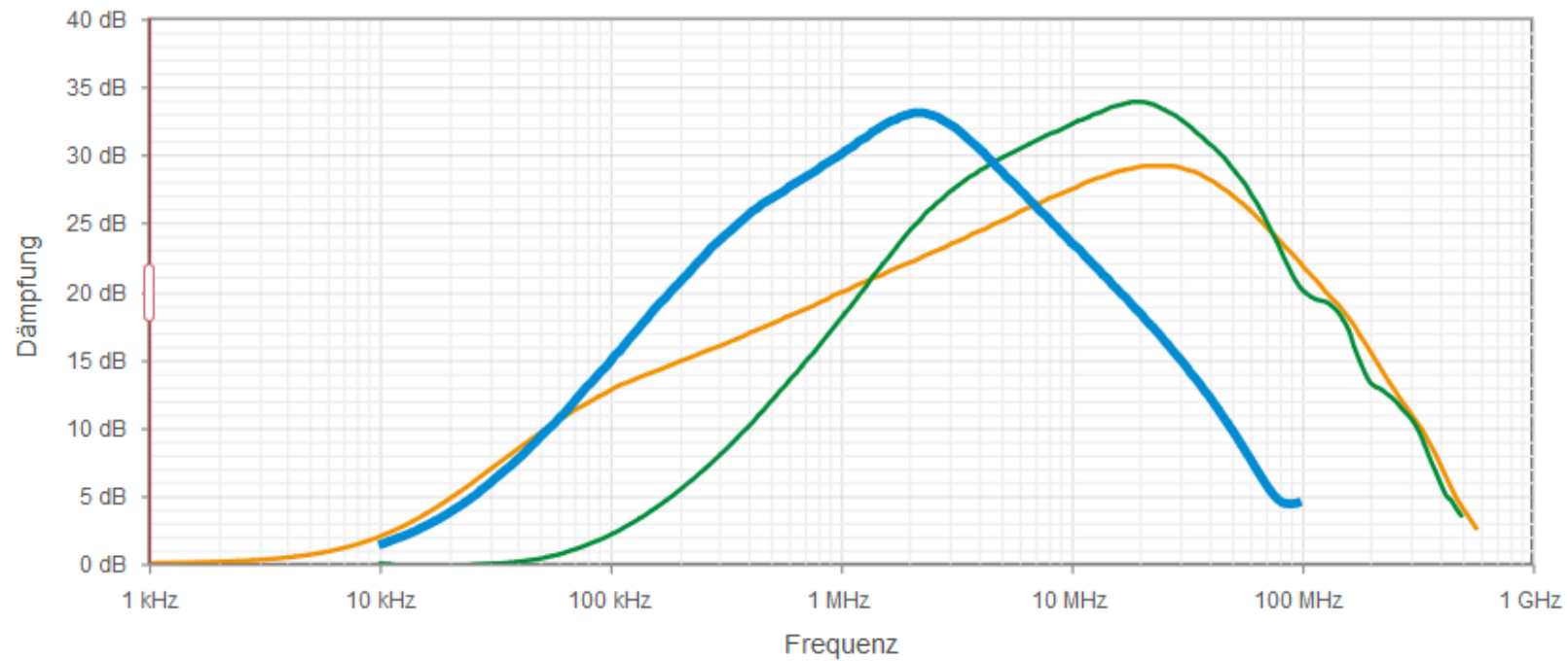
Gleichtakt Einfügedämpfung @50Ω
