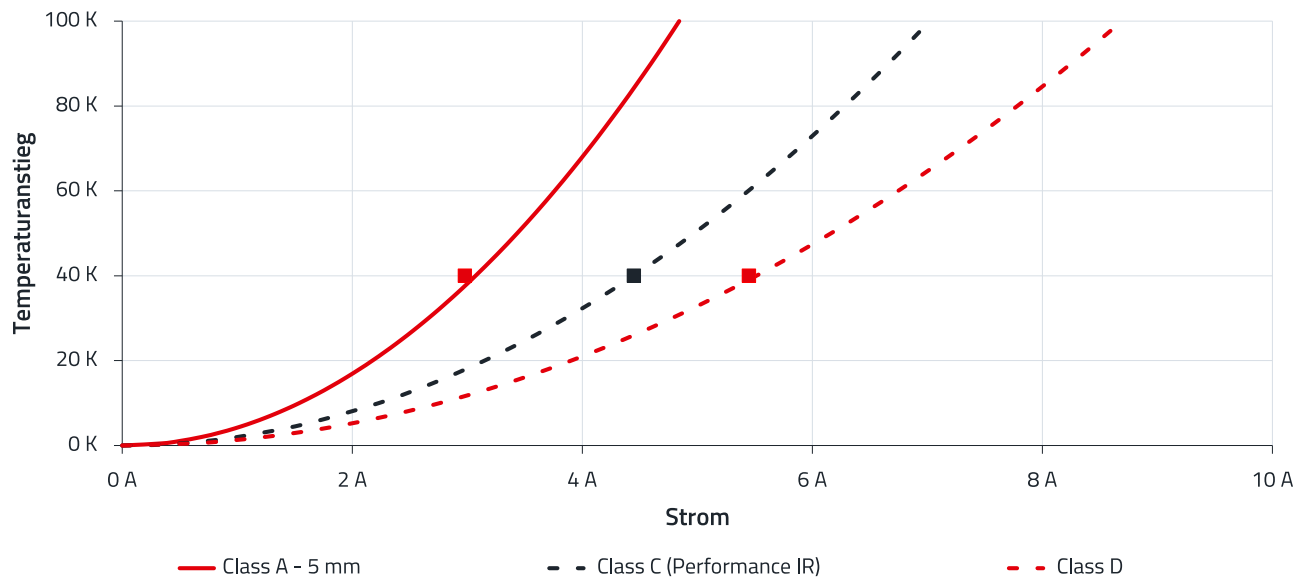
Abbildung 4: Vergleich der Eigenwärmerzeugung von WE-LHMI 744 373 460 68 auf verschiedenen IEC 62024-2-konformen Leiterplatten und dem unter Verwendung des Nennstromrechners berechneten Strom für einen Temperaturanstieg von 40 K (Datenpunkte)
