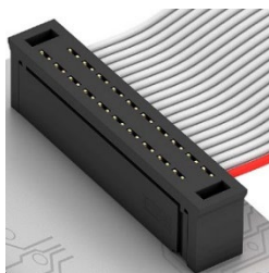
Abbildung 2: SKEDD Technologie spart Steckverbindersockel ein
