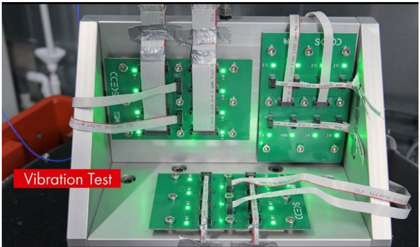
Abbildung 4: Testaufbau Vibrationstest
