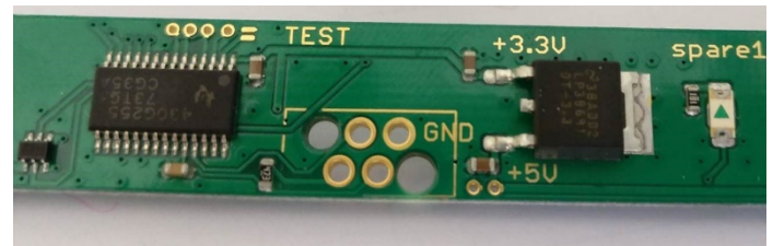
Abbildung 3: Layout und Platzbedarf auf der Leiterplatte
