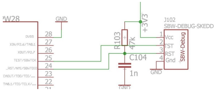
Abbildung 4: Pinbelegung des REDFIT IDC SKEDD als Debug-Stecker
