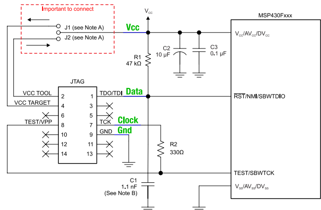
Abbildung 2: Debug-Leitungen und Stromversorgung im Schaltplan des TI-MSP430 (Quelle: TI MSP430 – Hardware Tools User's Guide Lit-No: SLAU278)
