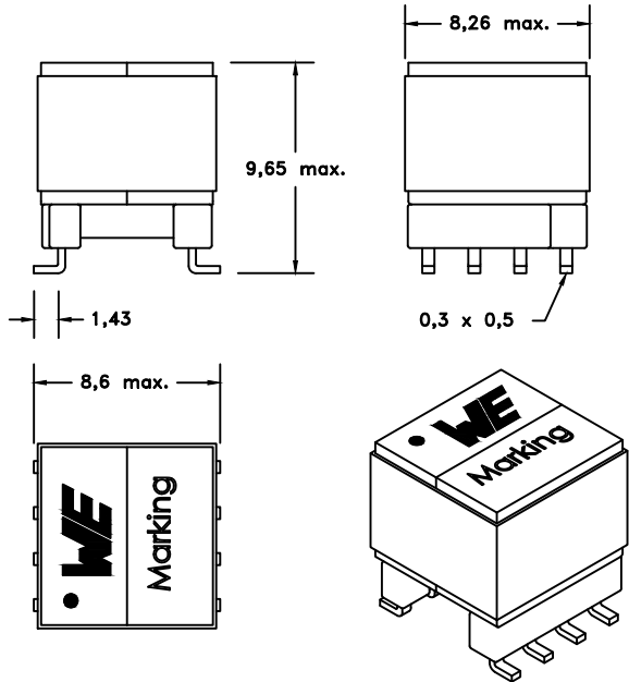
SCALE 3:1
