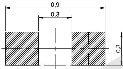
Scale - 50:1
