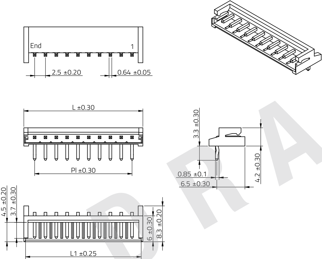
Scale-2:1
