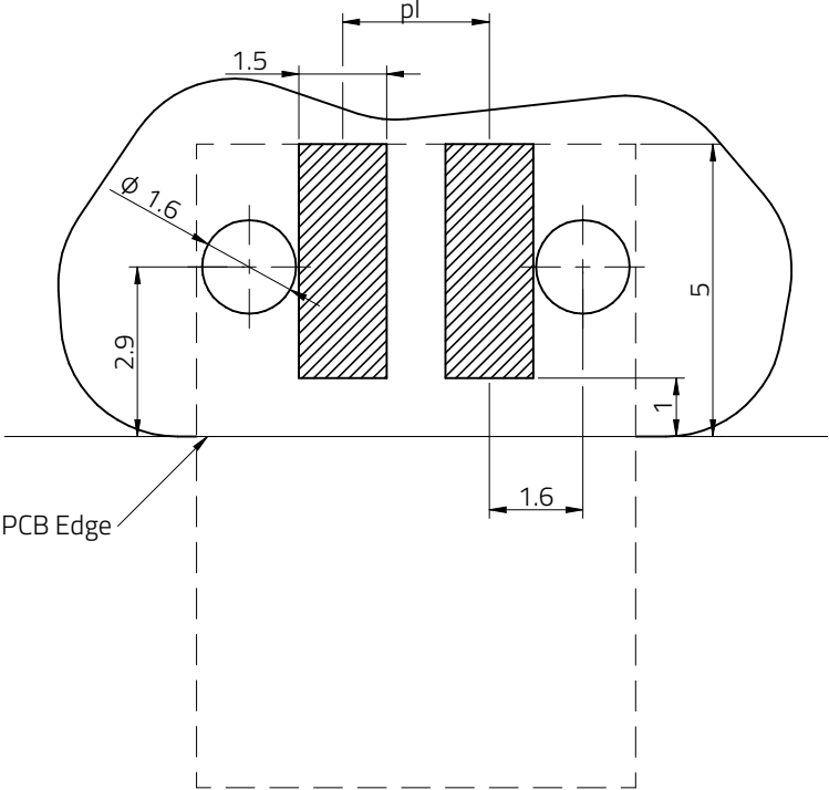
Scale - 4:1
