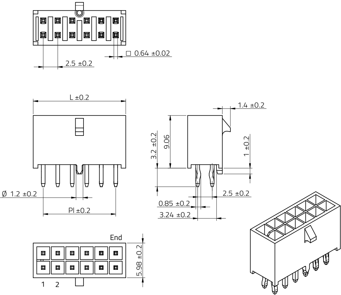
Scale - 2,5:1
