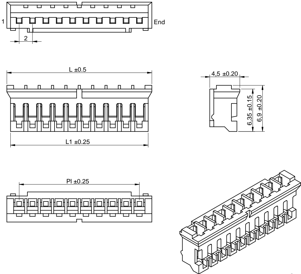
Scale - 3:1
