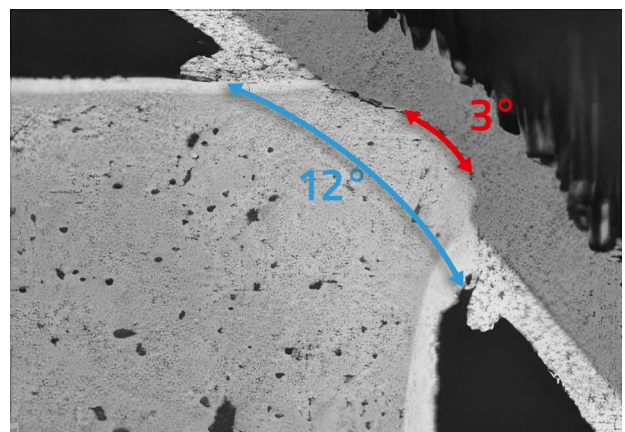
Abbildung 2: Erforderlicher Anschlussflächenwinkel von nur 3^\circ .
