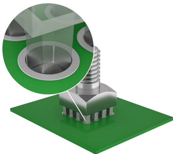
Abbildung 1: PRESS-FIT-Technologie.
