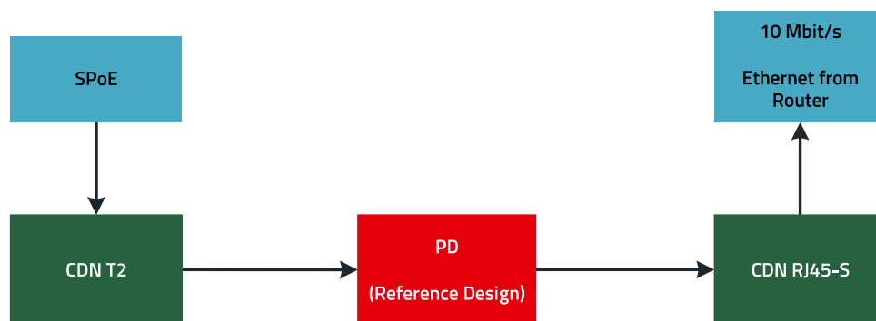
Abbildung 9: Prüfaufbau zur Prüfung der Funkstörspannung am PD.
