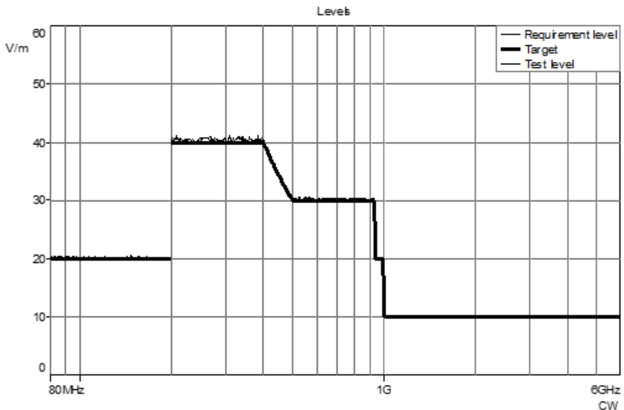
Abbildung 16: Maximaler Prüfpegel der gestrahlten Störfestigkeitsprüfung.
