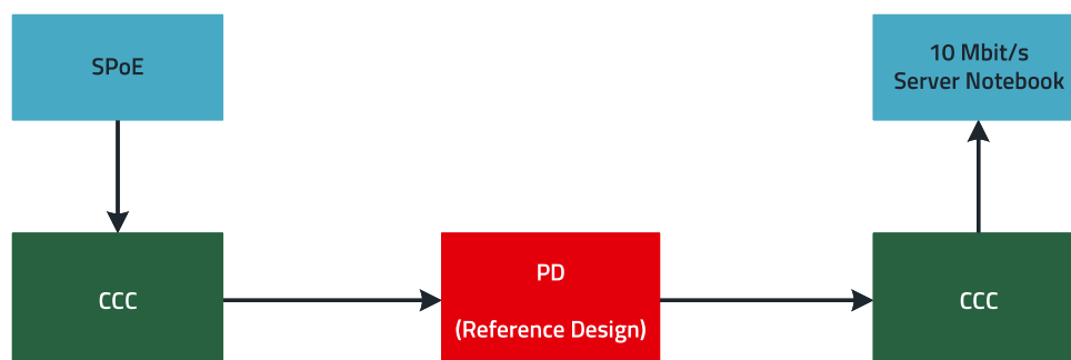
Abbildung 21: Prüfaufbau zur Prüfung der Störfestigkeit gegen Bursts am PD.
