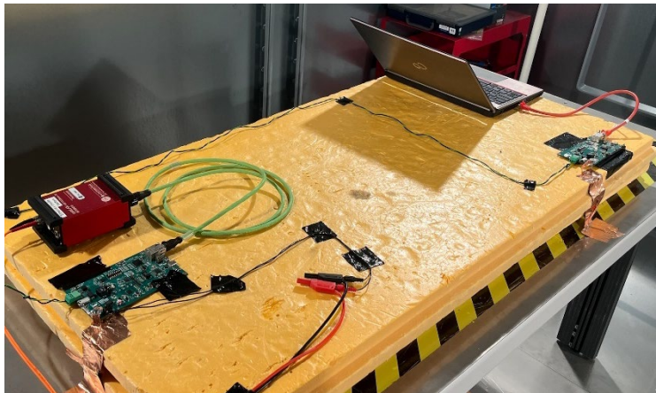
Abbildung 22: Im Bild links ist der Prüfaufbau des SPoE-Reference-Designs zur Prüfung gegen schnelle transiente Störgrößen dargestellt und im Bild rechts ist der Masseanschluss zu sehen.
