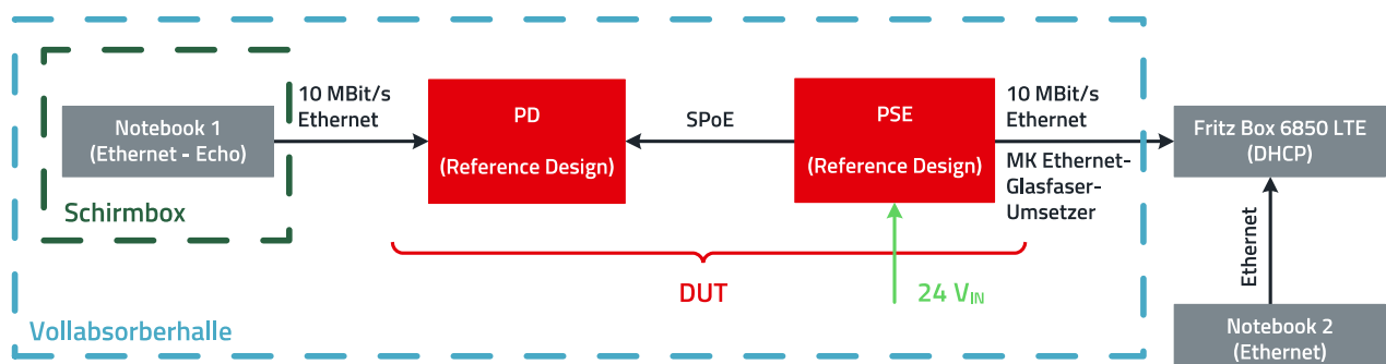
Abbildung 5: Blockdiagramm zur Prüfung der gestrahlten Störaussendung und Störfestigkeit.
