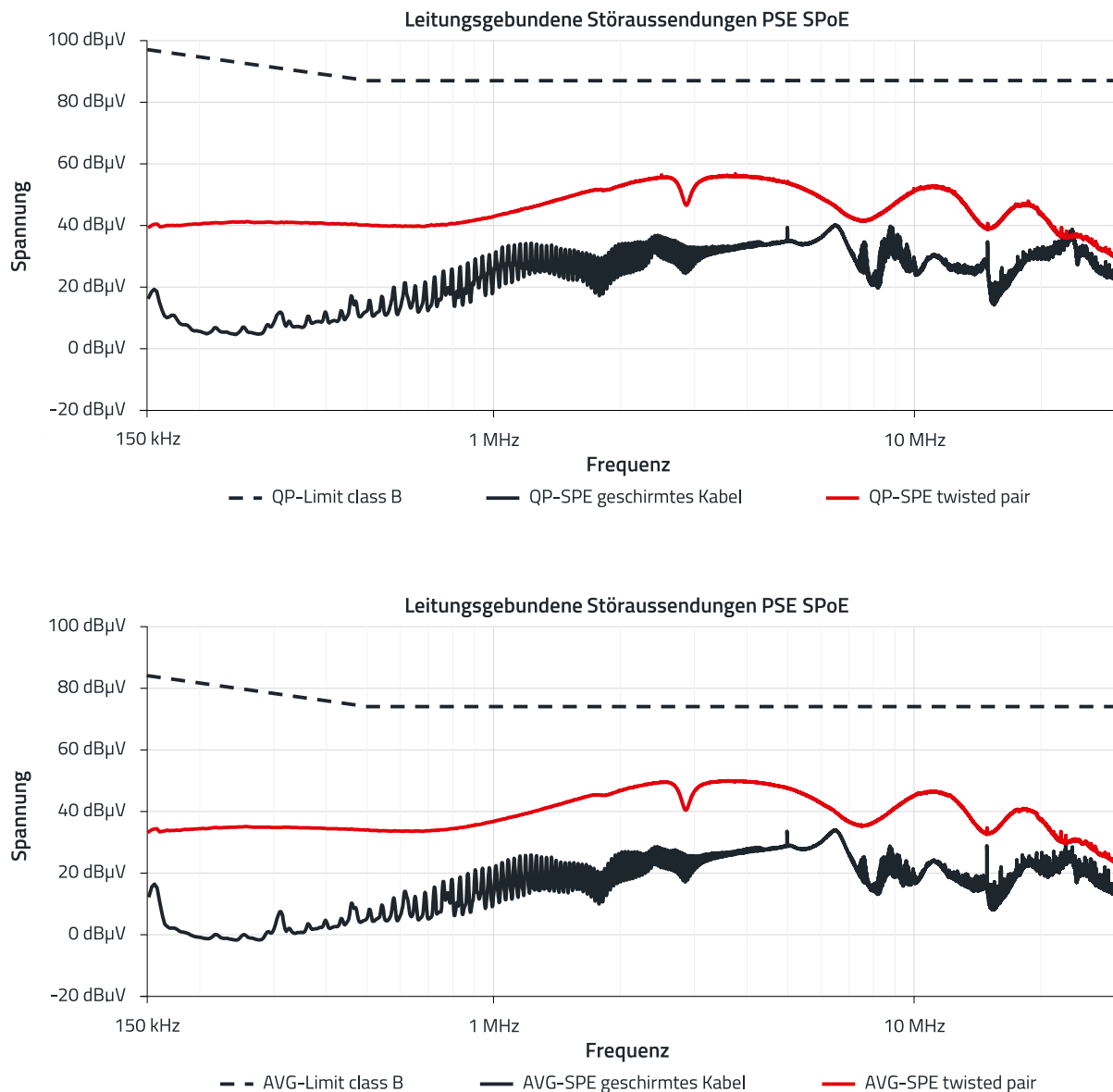
Abbildung 12: Ergebnisse der leitungsgeführten Störaussendung auf der SPoE-Schnittstelle des PSE. Oben sind die Ergebnisse des Quasipeakdetektors und unten die Ergebnisse des Mittelwertdetektors dargestellt.
