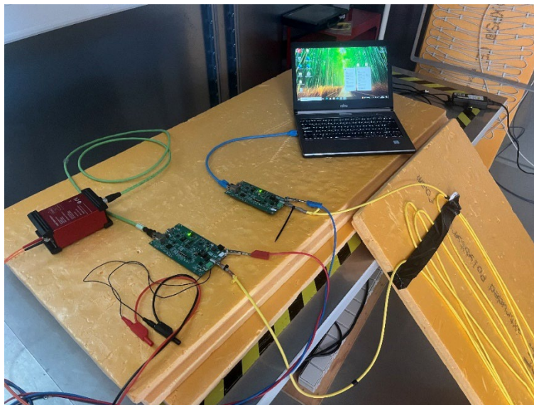
Abbildung 27: Surgeeinkopplung auf der geschirmten SPoE-Schnittstelle. Das PSE wird mittels Surge-CDN am Versorgungseingang (alternativ Batteriebetrieb) galvanisch von der Erde getrennt.
