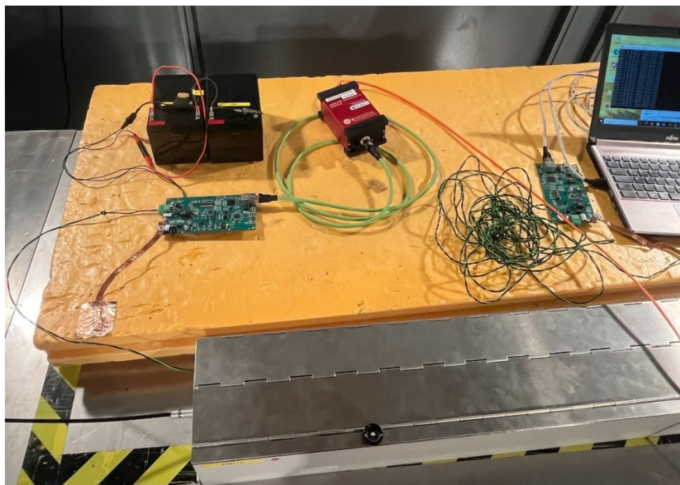
Abbildung 23: Burstprüfung mit der isoliert betrachteten SPoE-Schnittstelle.
