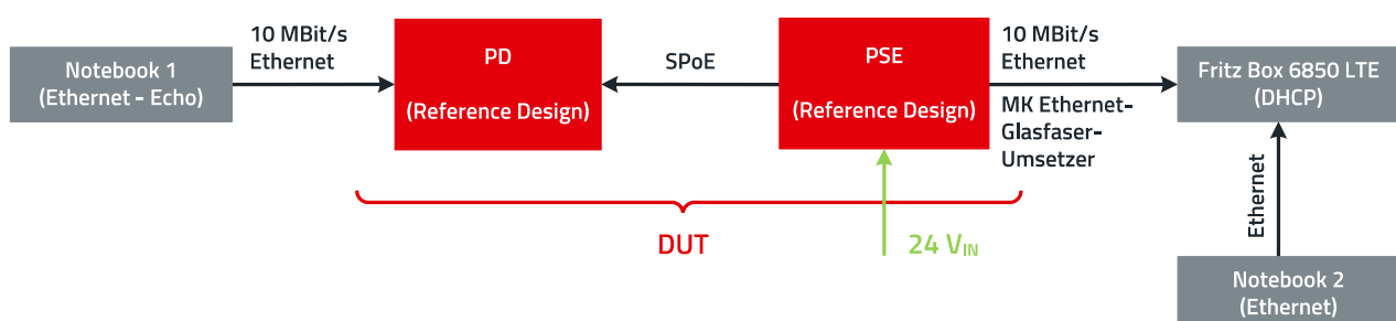
Abbildung 2: Prüfaufbau zur Performance-Evaluierung des SPoE-Reference-Designs.
