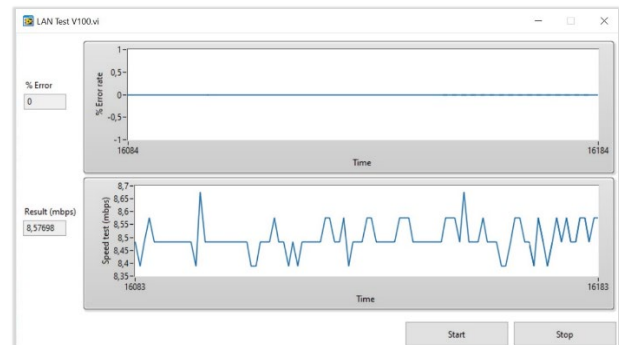
Abbildung 3: Monitoring der SPoE-Schnittstelle. PSE und PD sind mittels Ethernet-Schnittstelle im Netzwerk eingebunden.
