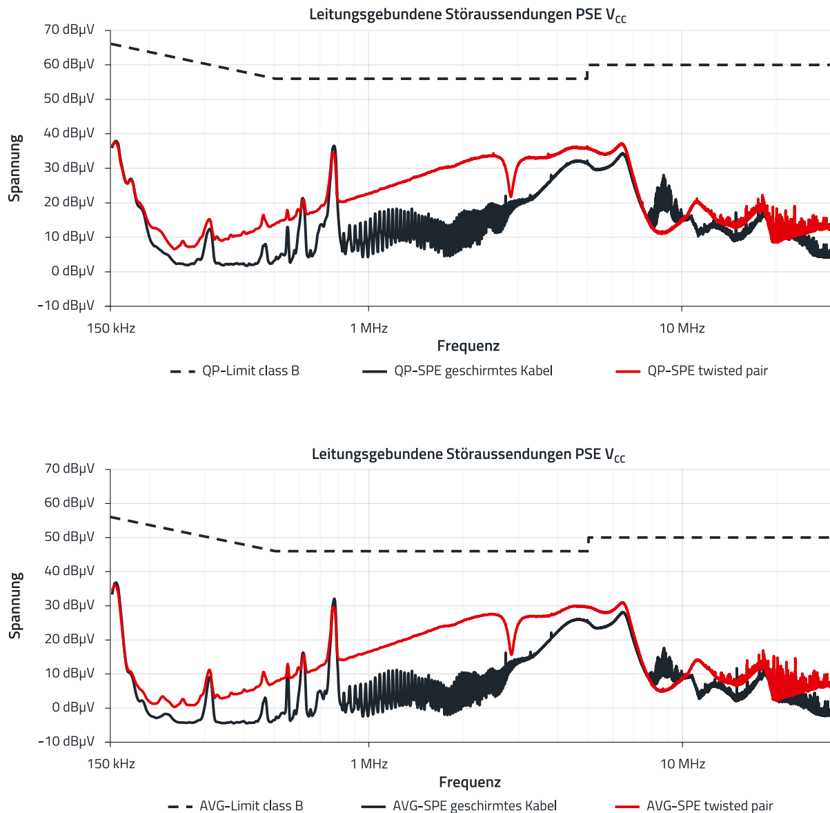
Abbildung 11: Ergebnisse der Funkstörspannungsmessung am DC-Port des PSE. Oben sind die Ergebnisse des Quasipeakdetektors und unten die Ergebnisse des Mittelwertdetektors dargestellt.
