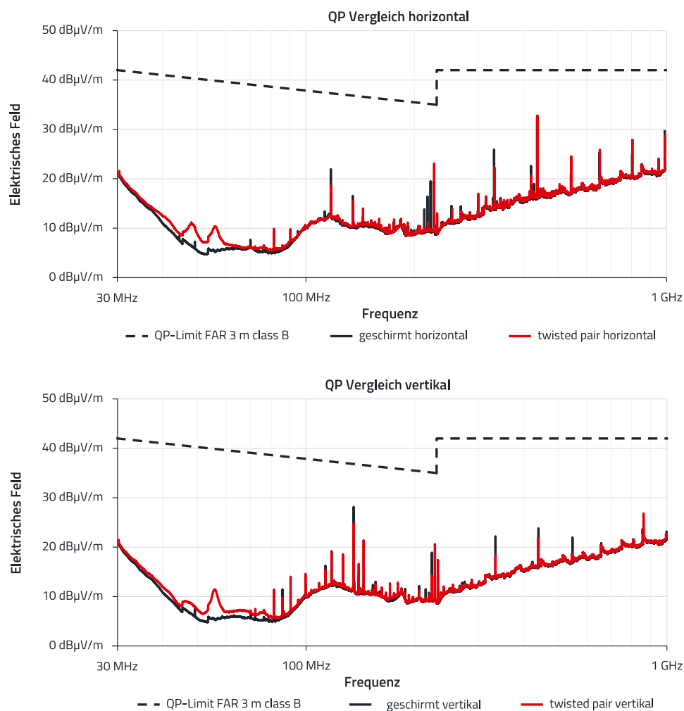
Abbildung 7: Vergleich der gestrahlten Störaussendung des SPoE-Reference-Designs bei Verwendung von geschirmter SPE-Leitung oder ungeschirmter Twisted-Pair-Leitung.
