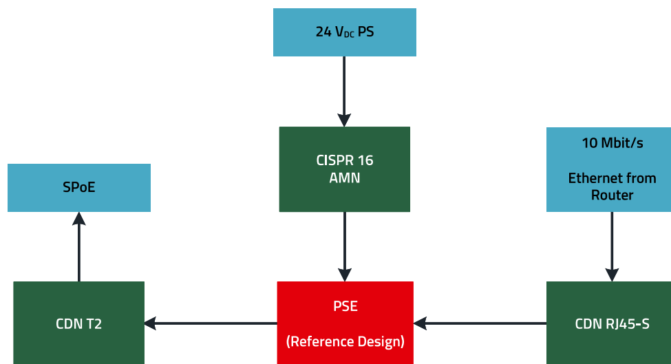
Abbildung 8: Prüfaufbau zur Prüfung der Funkstörspannung am PSE.
