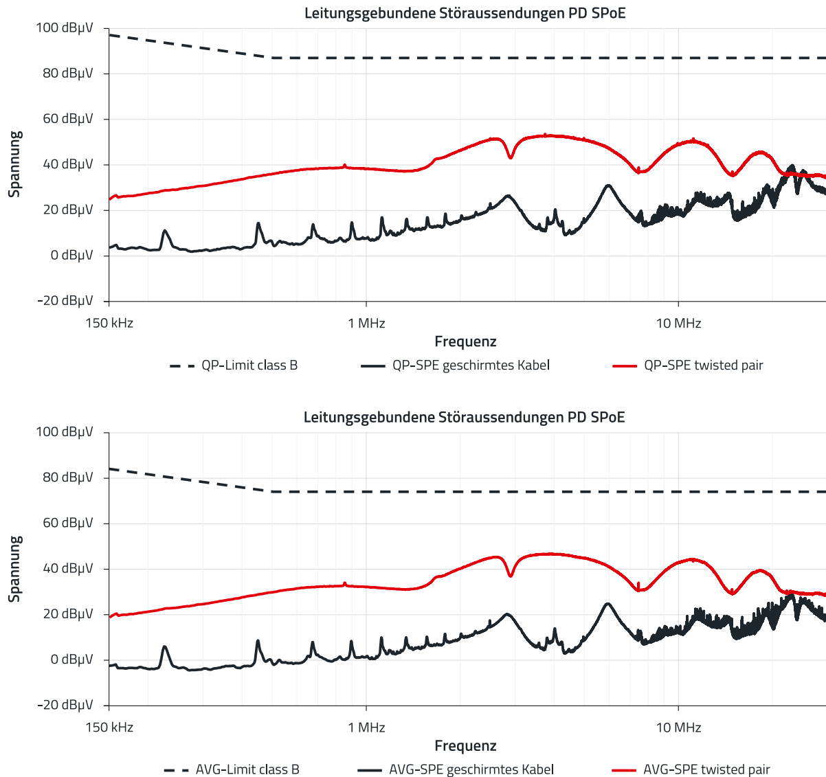
Abbildung 14: Ergebnisse der leitungsgeführten Störaussendung auf der SPoE-Schnittstelle des PD. Oben sind die Ergebnisse des Quasipeakdetektors und unten die Ergebnisse des Mittelwertdetektors dargestellt.
