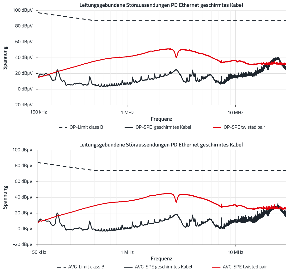
Abbildung 15: Ergebnisse der leitungsgeführten Störaussendung auf der Ethernet-Schnittstelle des PD bei Verwendung einer cat5e SF/UTP-Leitung. Oben sind die Ergebnisse des Quasipeakdetektors und unten die Ergebnisse des Mittelwertdetektors dargestellt.
