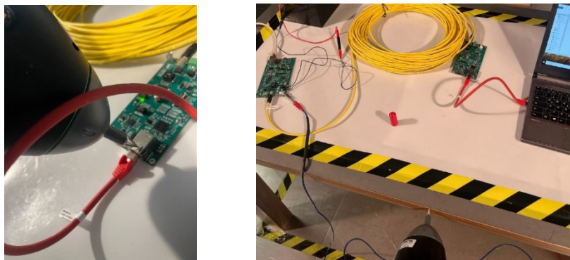
Abbildung 28: ESD-Prüfung des SPoE-Reference-Designs. Links: Kontaktentladung auf der geschirmten Ethernet-Buchse. Rechts: Indirekte ESD-Prüfung mittels Horizontaler Koppelplatte (HCP).
