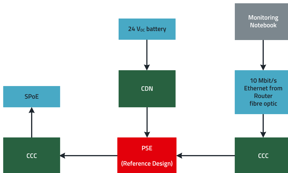
Abbildung 20: Prüfaufbau zur Prüfung der Störfestigkeit gegen Bursts am PSE.
