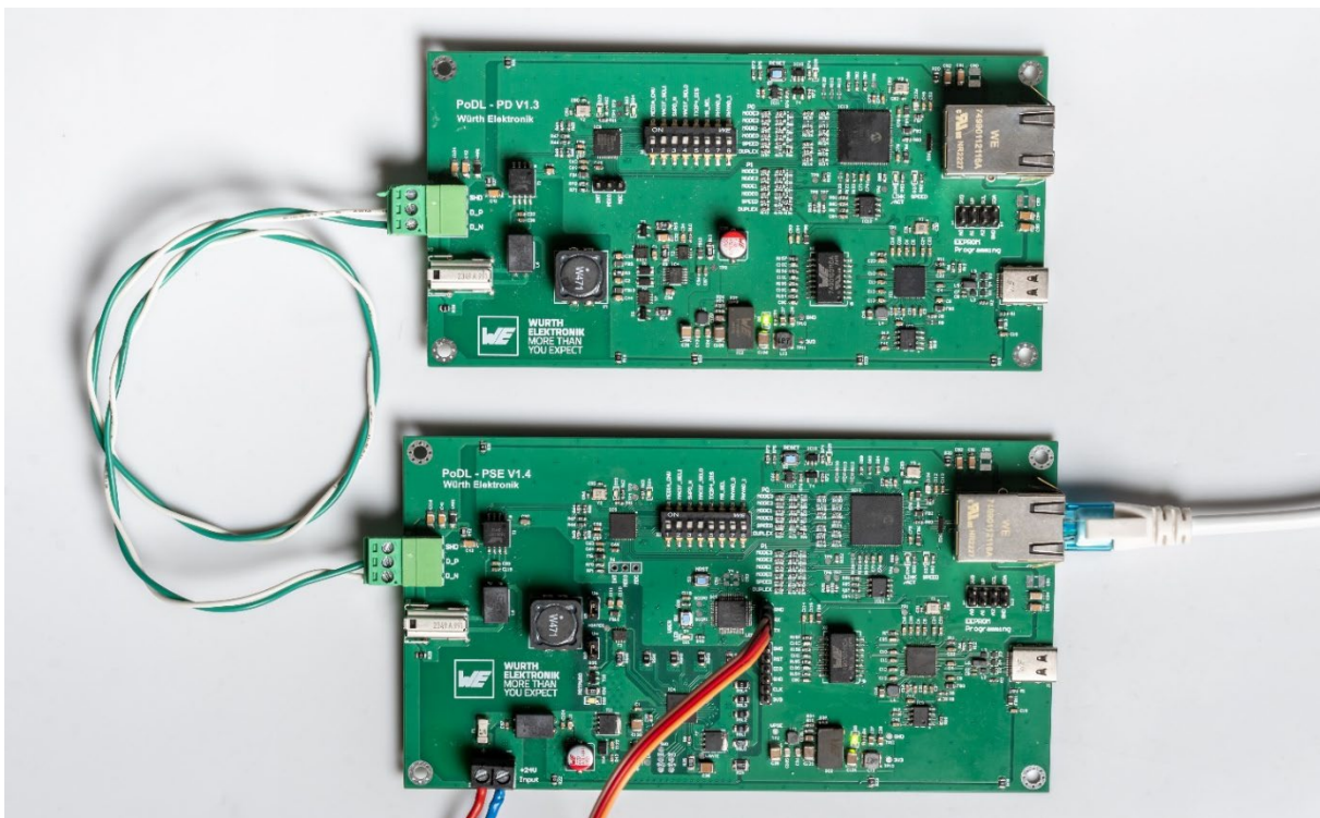
Abbildung 1: PSE (Board im Bild unten) und PD (Board im Bild oben) des RD041 bei der Inbetriebnahme.
