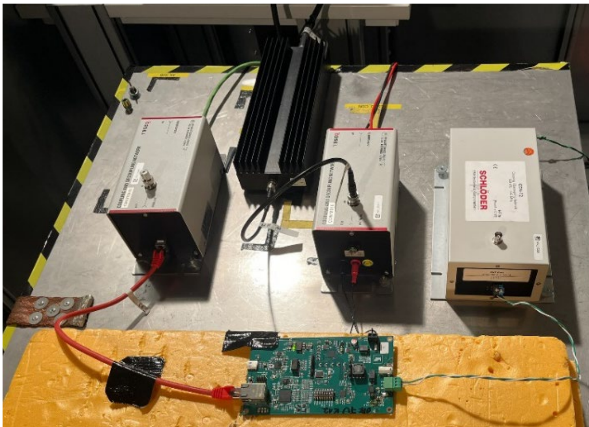
Abbildung 19: Leitungsgeführte Störfestigkeitsprüfung des PSE-Boards.
