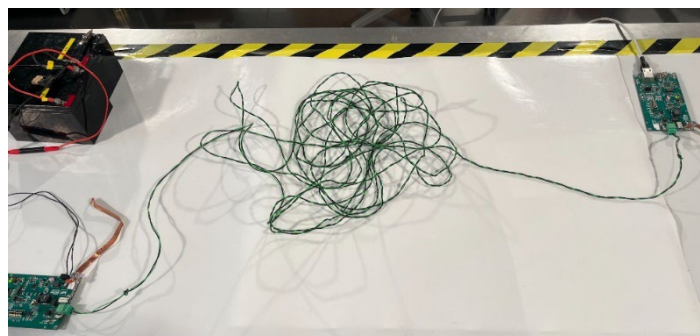
Abbildung 29: ESD-Prüfung des SPoE-Reference-Designs bei Verwendung einer ungeschirmten Twisted-Pair-Leitung.
