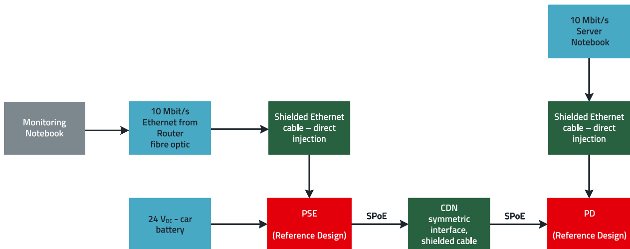
Abbildung 26: Prüfaufbau zur Prüfung der Störfestigkeit gegen Surgepulse. Die Ethernet-Schnittstelle wird galvanisch getrennt betrieben.
