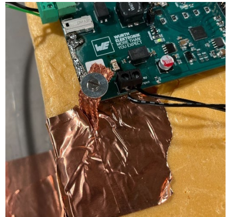
Abbildung 22: Im Bild links ist der Prüfaufbau des SPoE-Reference-Designs zur Prüfung gegen schnelle transiente Störgrößen dargestellt und im Bild rechts ist der Masseanschluss zu sehen.
