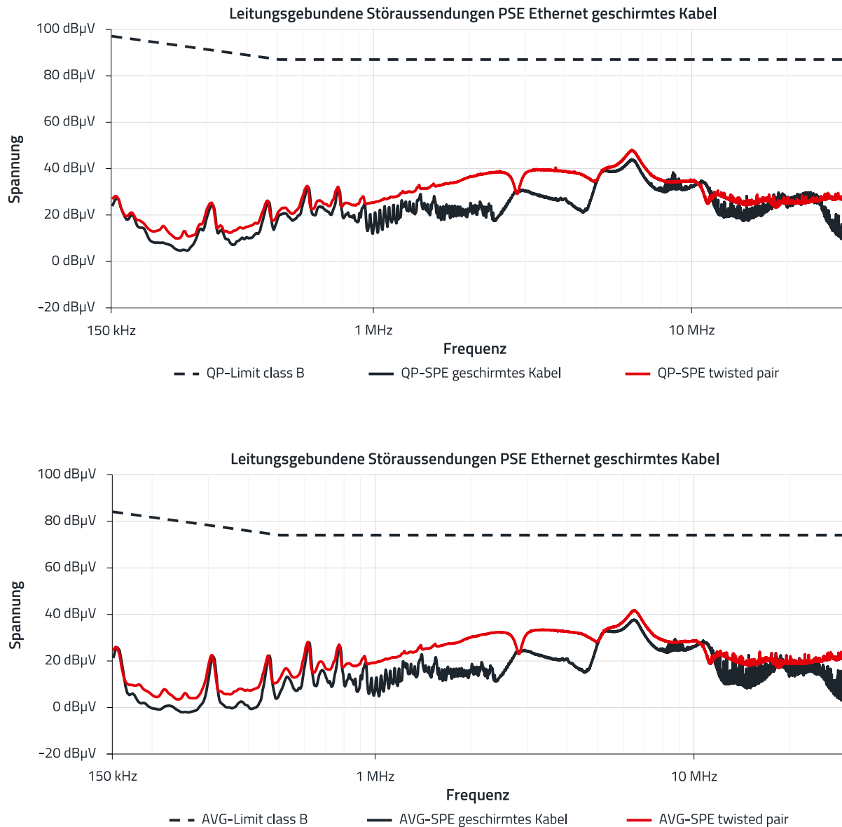
Abbildung 13: Ergebnisse der leitungsgeführten Störaussendung auf der Ethernet-Schnittstelle des PSE bei Verwendung einer cat5e SF/UTP-Leitung. Oben sind die Ergebnisse des Quasipeakdetektors und unten die Ergebnisse des Mittelwertdetektors dargestellt.
