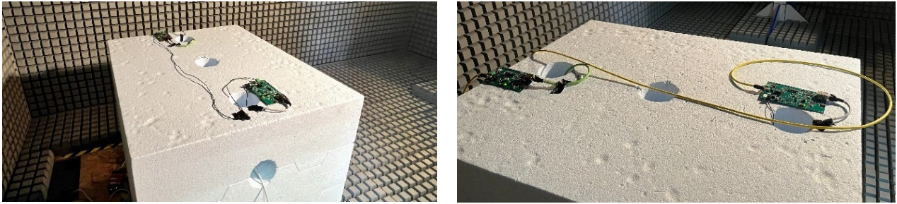
Abbildung 6: Prüfung der gestrahlten Störaussendung des SPoE-Reference-Designs in der Vollabsorberhalle.
