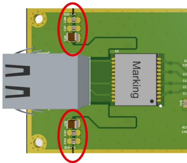
Abbildung 4: Schirmanbindung der Ethernet-Buchse nach ANP116. Auf jeder Seite ein MLCC, der Varistor ist im Bild nicht eingezeichnet.
