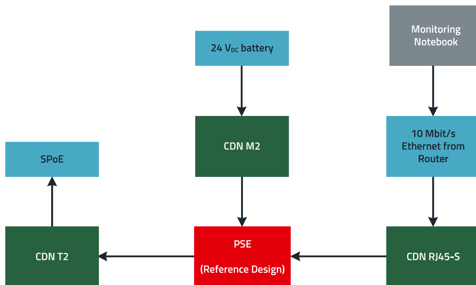
Abbildung 17: Prüfaufbau zur Prüfung der leitungsgeführten Störfestigkeit am PSE.
