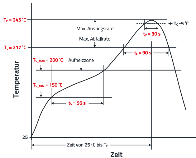
Abbildung 11: Benutztes Reflow-Profil zur Qualifizierung von WE THR-Produkten.
