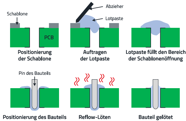
Abbildung 12: Schematischer Ablaufplan des Reflow Prozesses.
