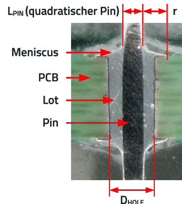
Abbildung 6: Darstellung einer guten Durchgangslötstelle.
