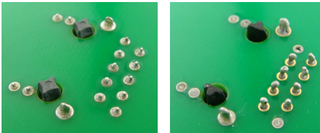
Abbildung 3: Perfektes Lötgergebnis mit sichtbarem Meniskus auf der linken Seite und schlechtes Lötgergebnis mit Lotkugeln auf der Oberseite der Pins aufgrund der zu großen Pinlänge.
