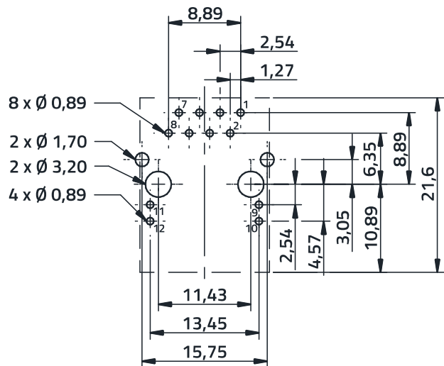
Abbildung 8: Empfohlenes Löttaugenmuster aus dem Datenblatt von WE-RJ45 THR 74980104400 .
