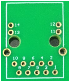
Abbildung 9: Platinen Layout.
