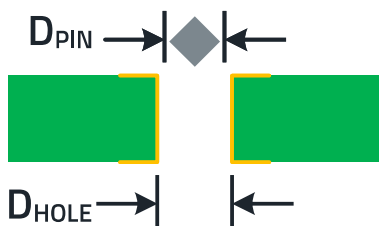
Abbildung 7: Designregel für den Durchmesser der Leiterplattenbohrung D_{HOLE} = D_{PIN} + 0,3 \text{ mm} .
