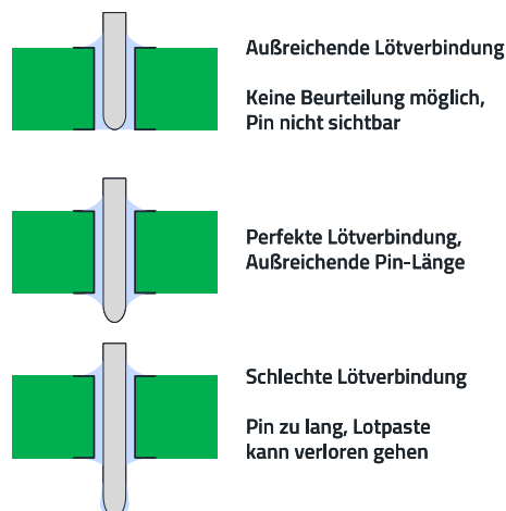
Abbildung 4: Das Lötgergebnis bei unterschiedlichen Pin-Längen.
