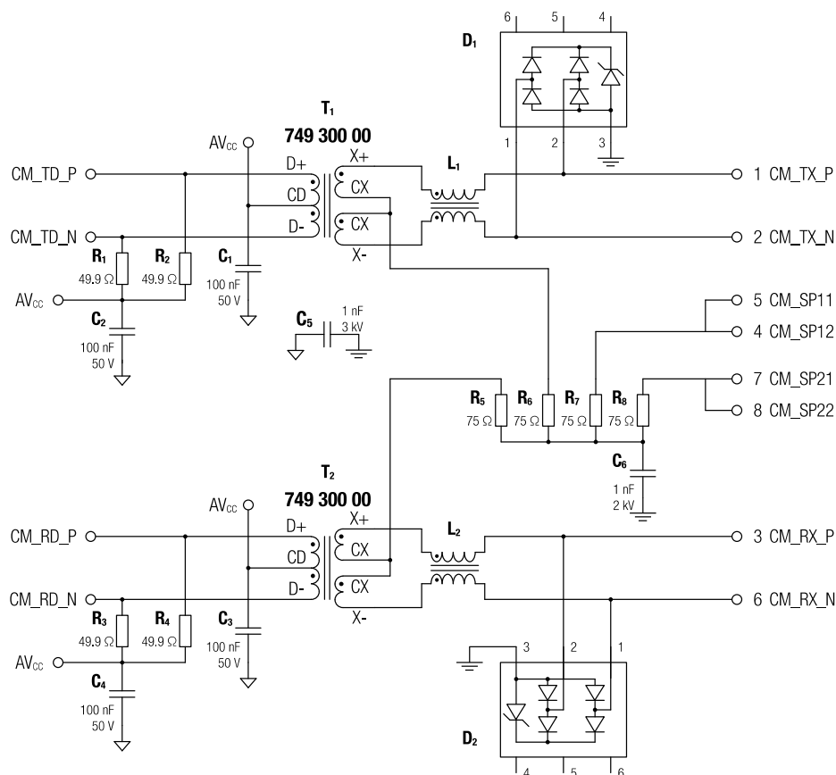
Abbildung 4: Schaltschema mit stromgesteuertem PHY
