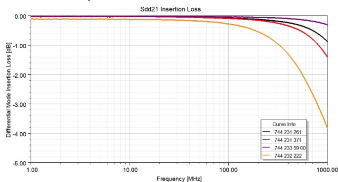
Abbildung 3: Vergleich der Differentiellen Einfügedämpfung (sdd21)
