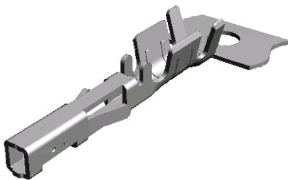
Abbildung 2: Der Standard-Crimp-Kontakt verfügt über eine starre Kontakthülse.
