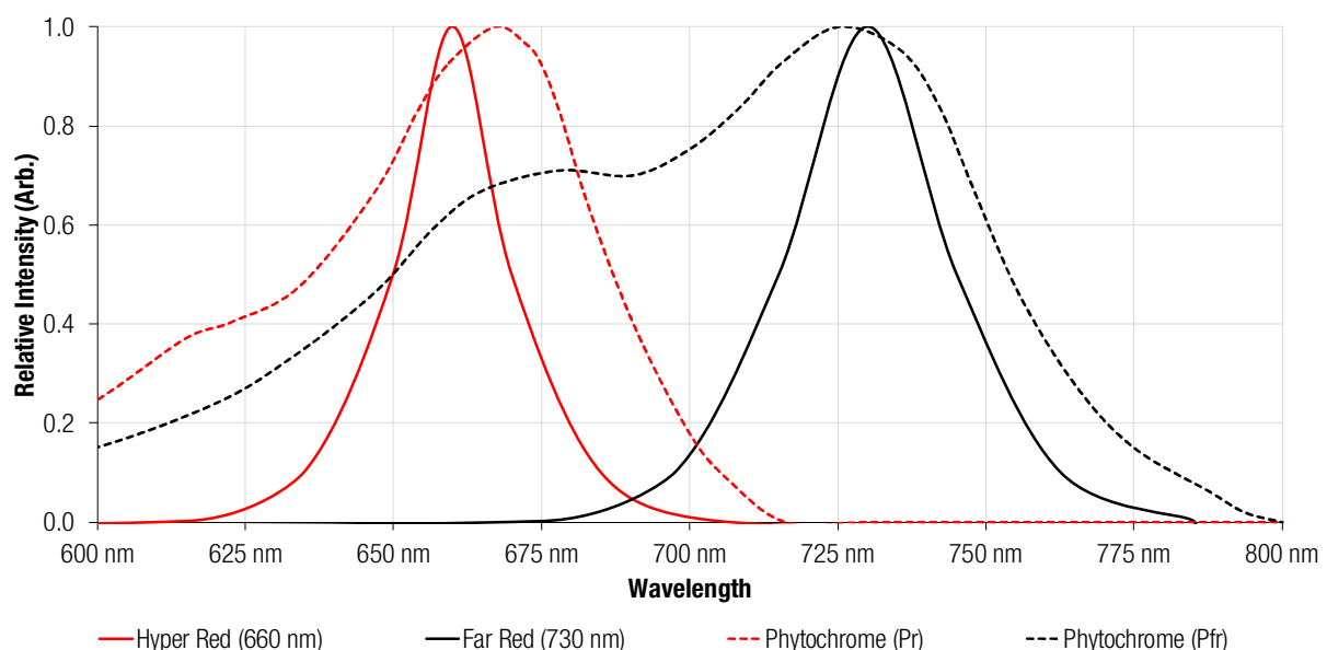
Abbildung 5: Die Absorptionsspektren von den Phytochromen Pr und Pfr und die Lichtleistung von den WL-SMDC hyperroten ( 150353HS74500 ) und dunkelroten ( 150353FS74500 ) keramischen LEDs.
