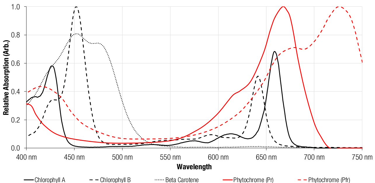
Abbildung 1: Typische Absorptionsspektren der Hauptpigmente von Pflanzen
