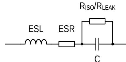
Abbildung 1: Ersatzschaltbild eines realen Kondensators
