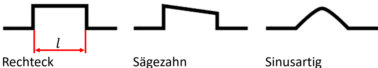
Abbildung 2: Mögliche Impulsformen im Einschaltmoment
