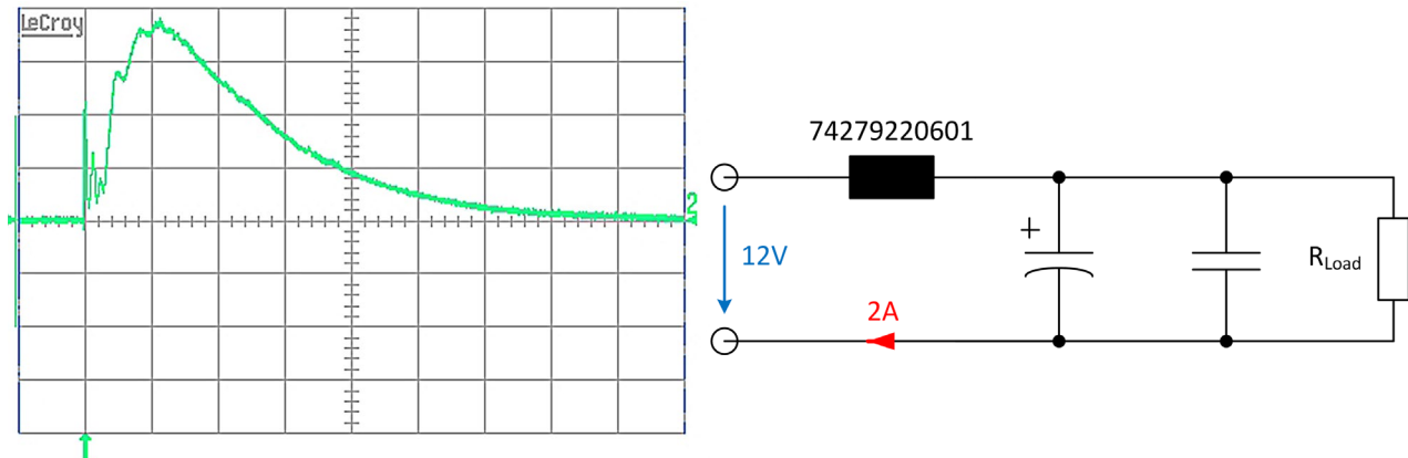
Abbildung 1: Anwendung mit Spitzenstrom im Einschaltmoment (5A/DIV | 100µs/DIV)
