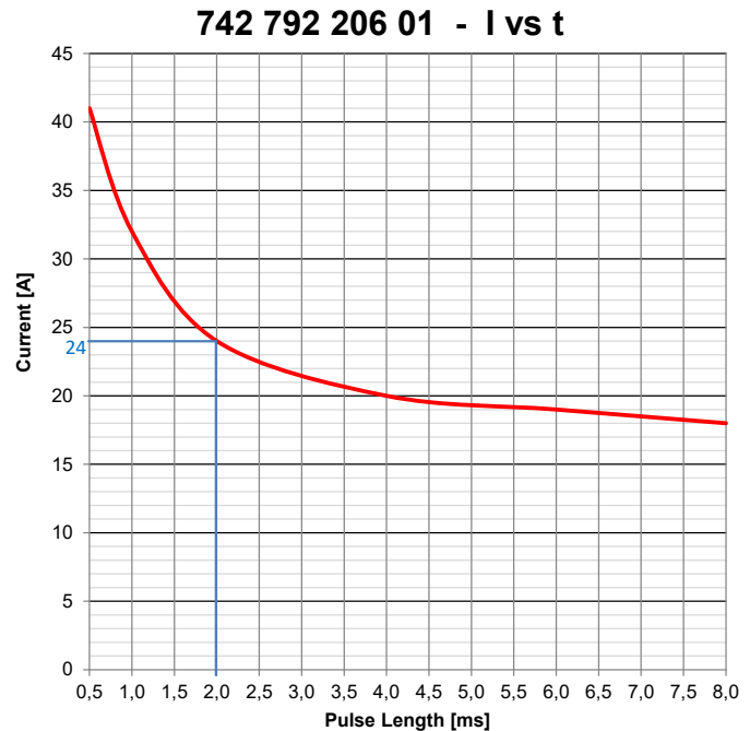
Abbildung 3: Spezifizierte Spitzenstrombelastbarkeit
