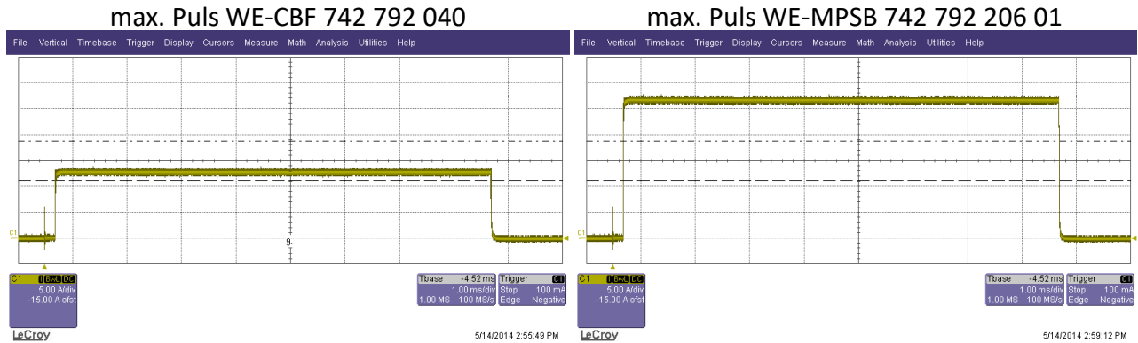
Abbildung 6: Pulsbelastbarkeit der WE-CBF und WE-MPSB-Serie im Vergleich
