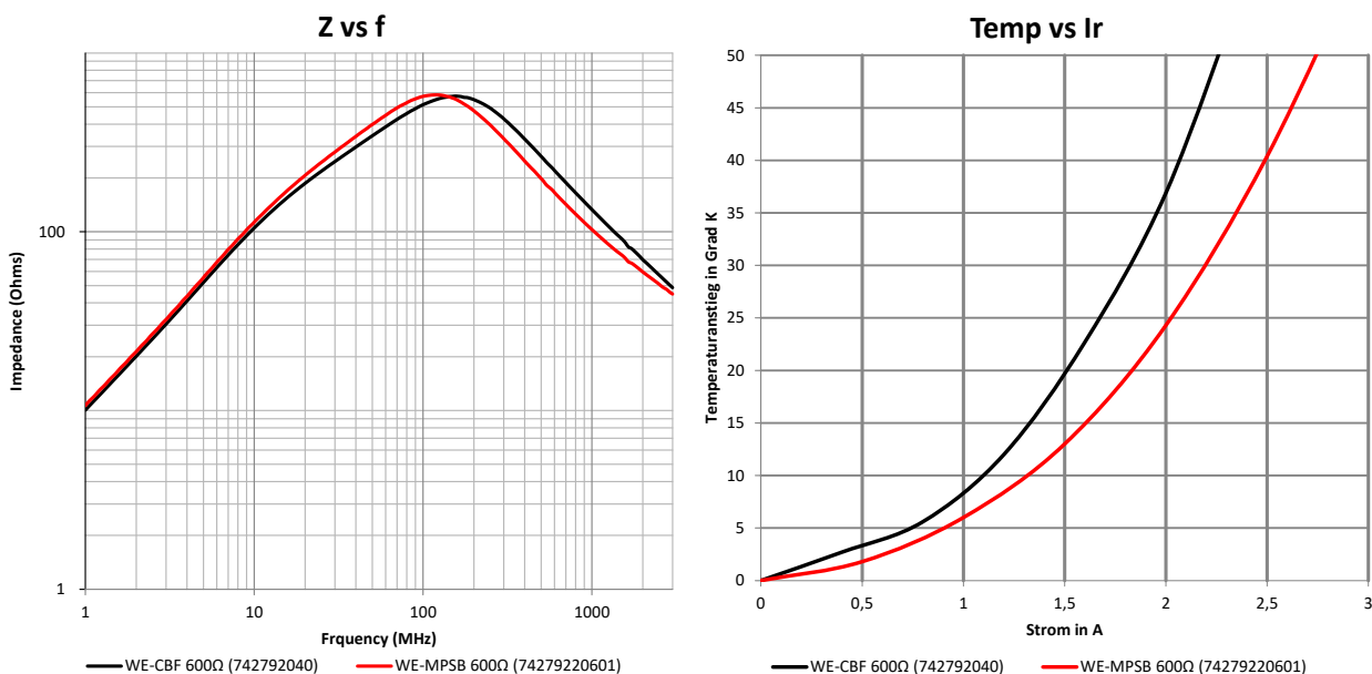
Abbildung 5: Vergleich der Impedanz und Nennstrombelastbarkeit des WE-CBF- und WE-MPSB-600- \Omega -Typs
