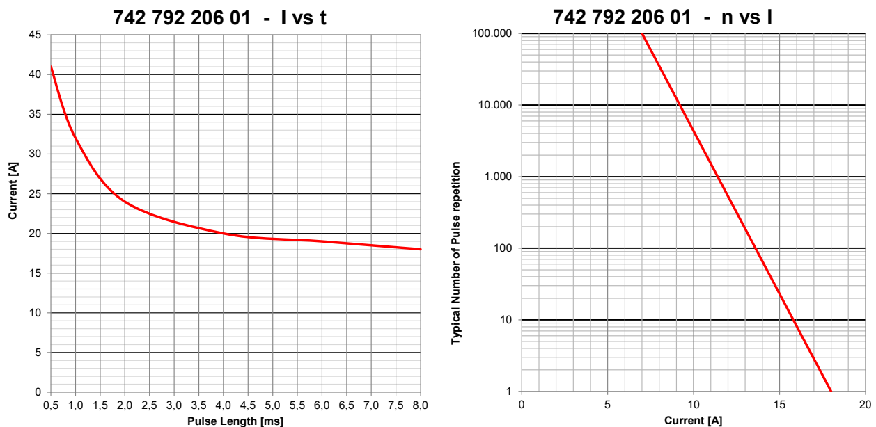
Abbildung 4: Darstellung des Stromes als Abhängigkeit zur Pulslänge und der Anzahl der Pulse bei 8 ms
