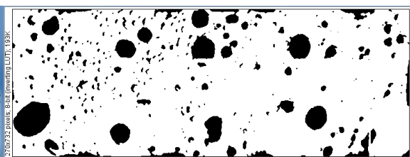
Abbildung 14 : Voidflächenberechnung für Abbildung 11 (linkes Pad)
