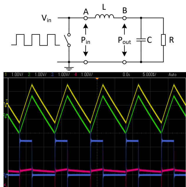
Abbildung 3: Aufbau des DC-DC-Wandlers zur Verlustbestimmung und resultierende Aufnahmen
