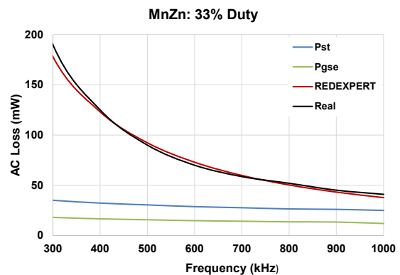
Abbildung 7: Drossel aus MnZn bei 33 % DC
