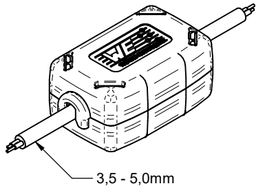
Scale - 1:1,25
