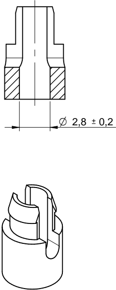
Scale- 5:1
